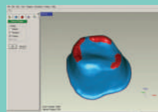
CAD/CAM analiza preparacije zuba izvedena na KaVo Everest sustavu.
